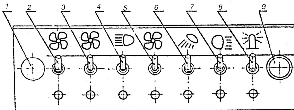
Рис. 8 Блок выключателей
