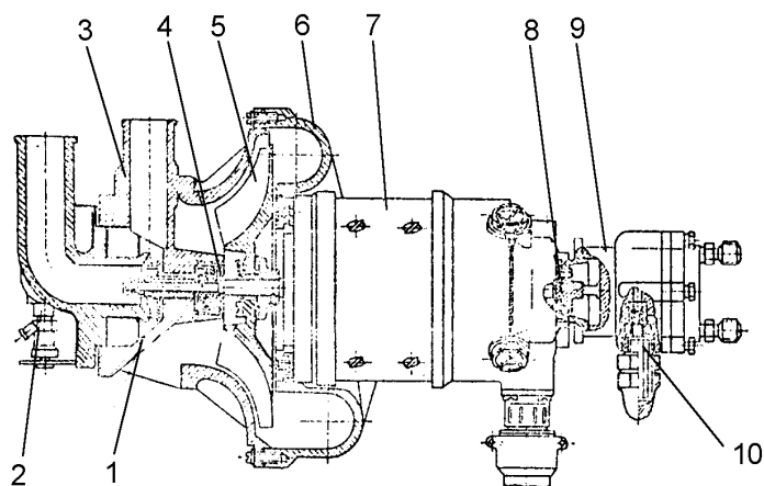
Рис. 27 Насосный агрегат
