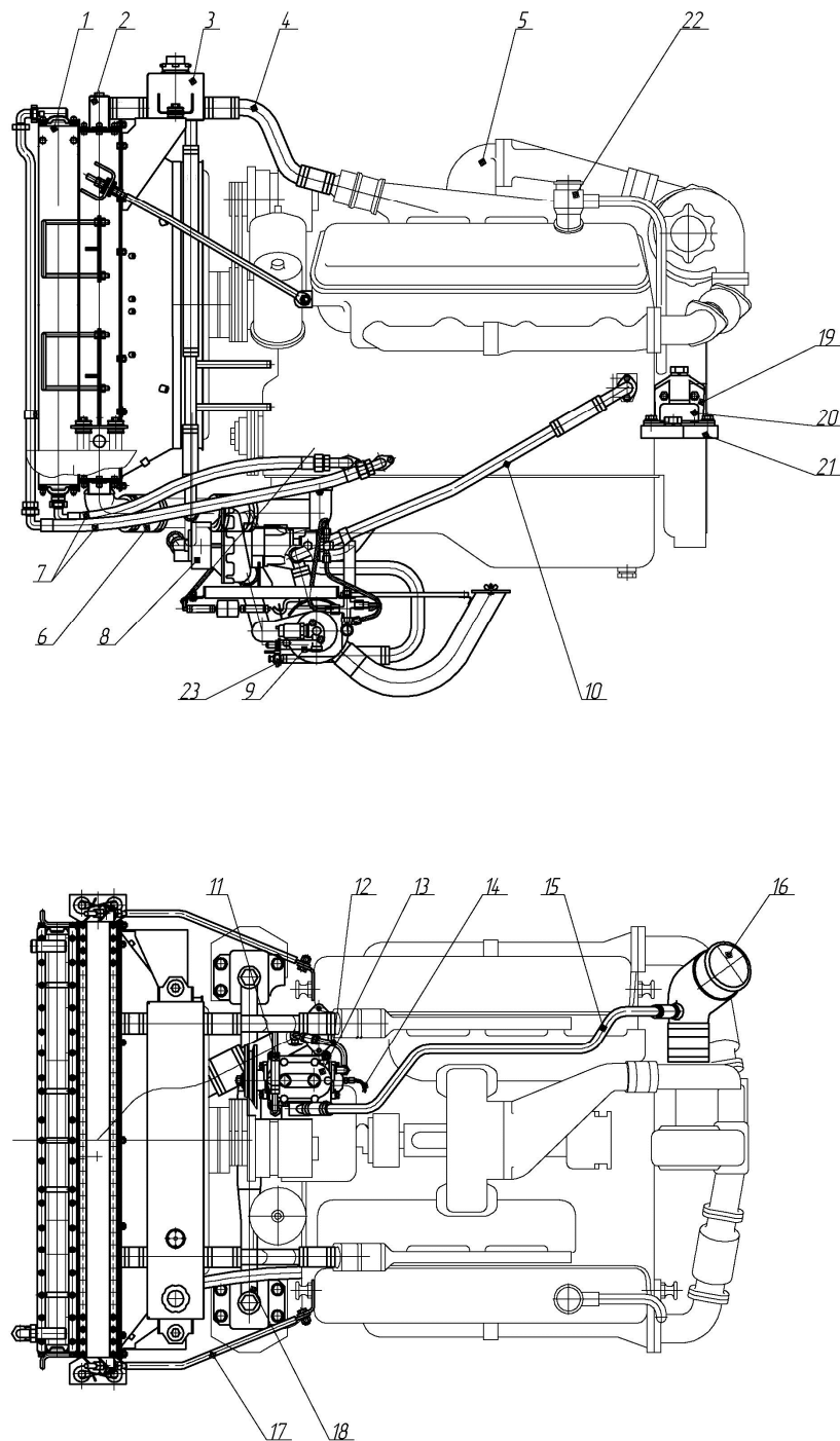
Рис. 21 Двигатель с системами
