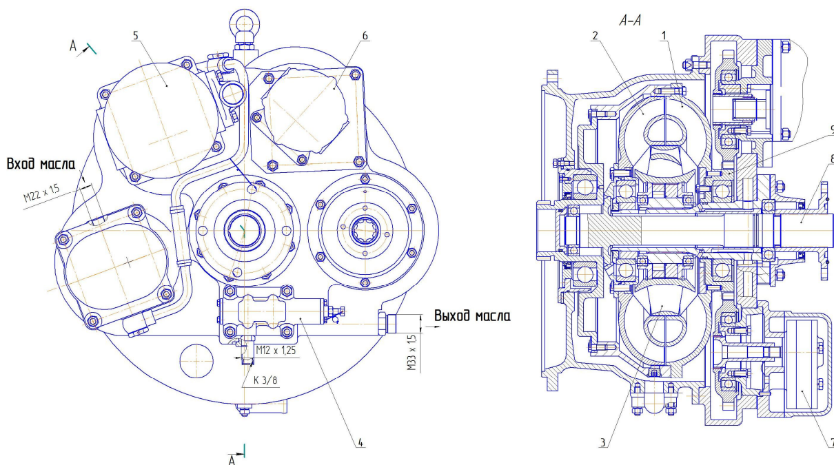
Рис. 30 Гидротрансформатор
