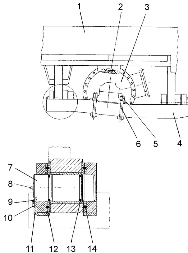
Рис. 56 Балансирная подвеска подмоторного моста
