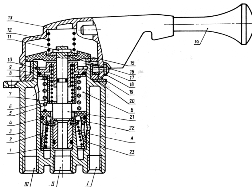
Рис. 52 Тормозной кран обратного действия с ручным управлением
