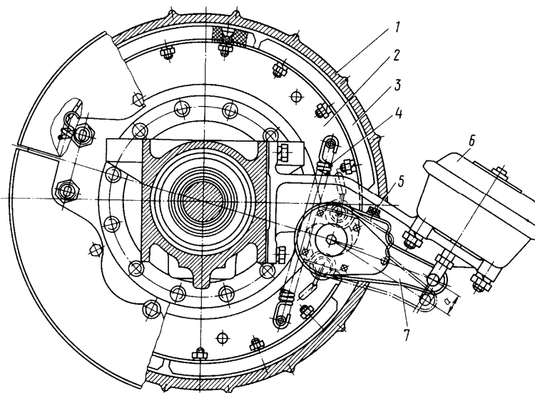
Рис. 71 Рабочий тормоз
