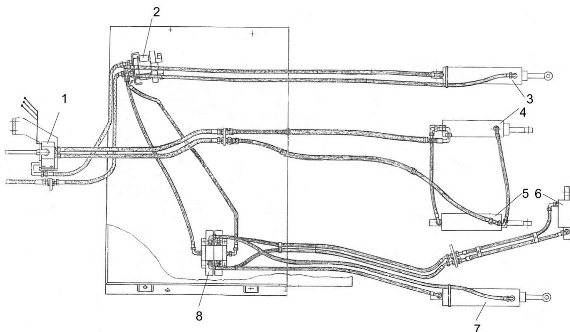
Рис. 44 Гидросистема рабочего оборудования бульдозера
