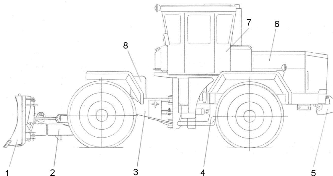
Рис. 1 Общий вид бульдозера К-702МБА-01-БКУ
