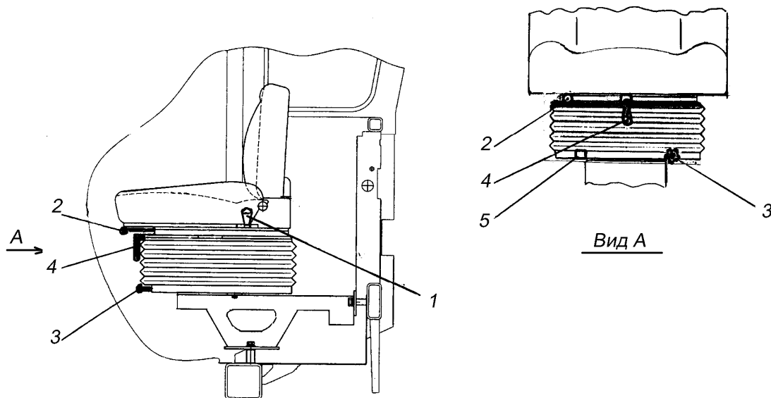
Рис. 54 Сиденье водителя
