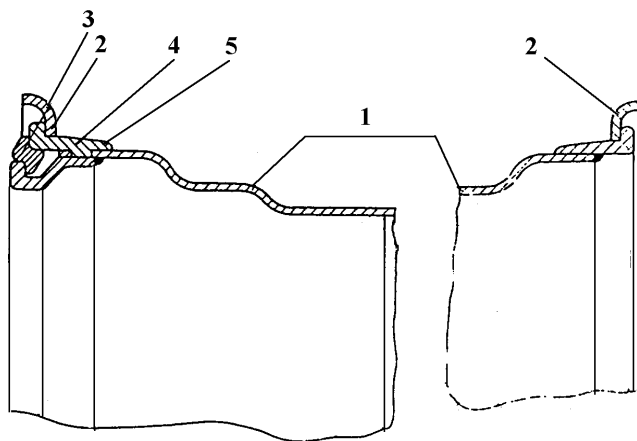
Рис. 59 Колесо дисковое разборное
