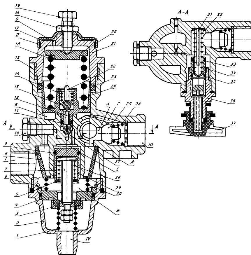
Рис. 50 Регулятор давления
