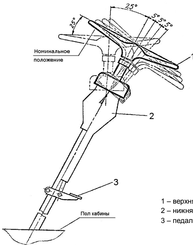
Рис. 14 Рулевая колонка
