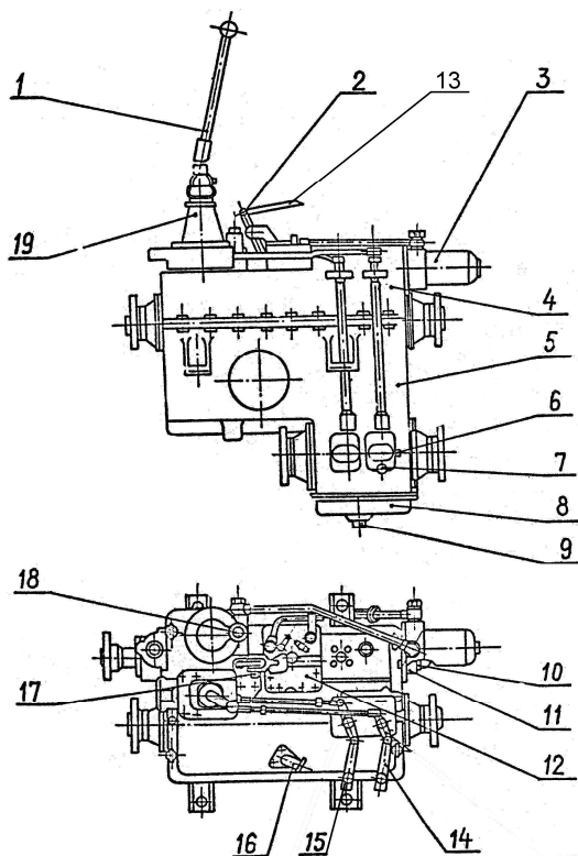
Рис. 31 Коробка передач
