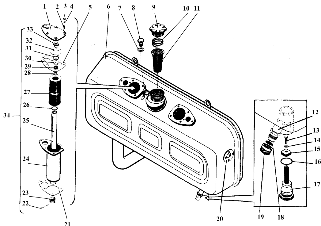
Рис. 74 Гидробак
