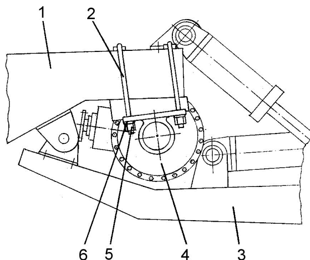
Рис. 57 Подвеска грузового моста
