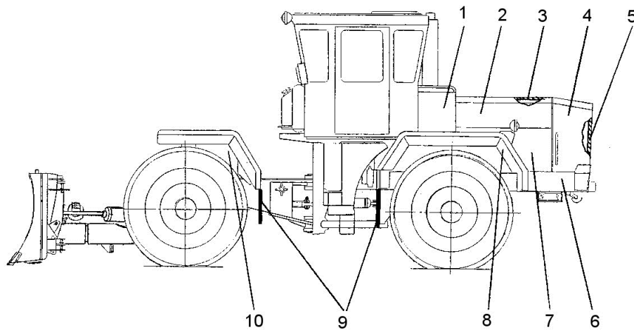
Рис. 60 Облицовка
