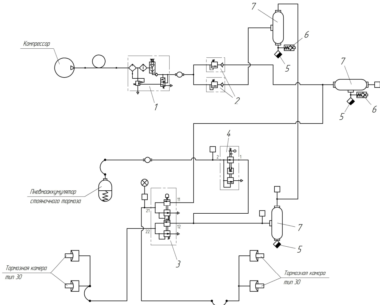
Схема пневмосистемы бульдозера
