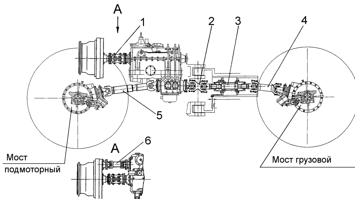
Рис. 40 Передача карданная
