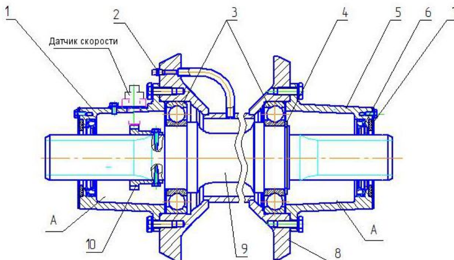
Рис. 41 Опора промежуточная
