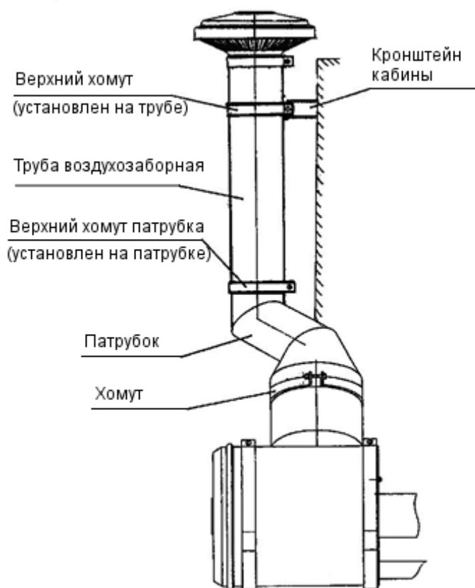
Рис. 15 Установка воздухозаборной трубы на машину
