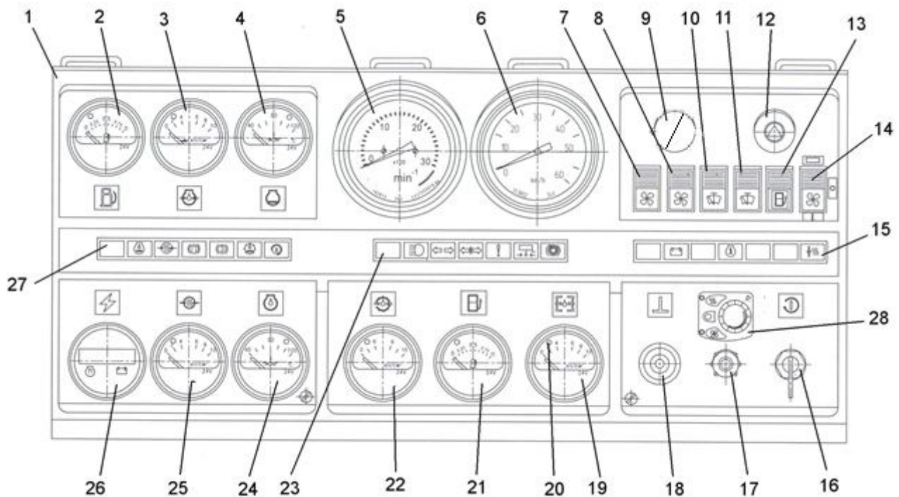
Рис. 3 Щиток приборов
